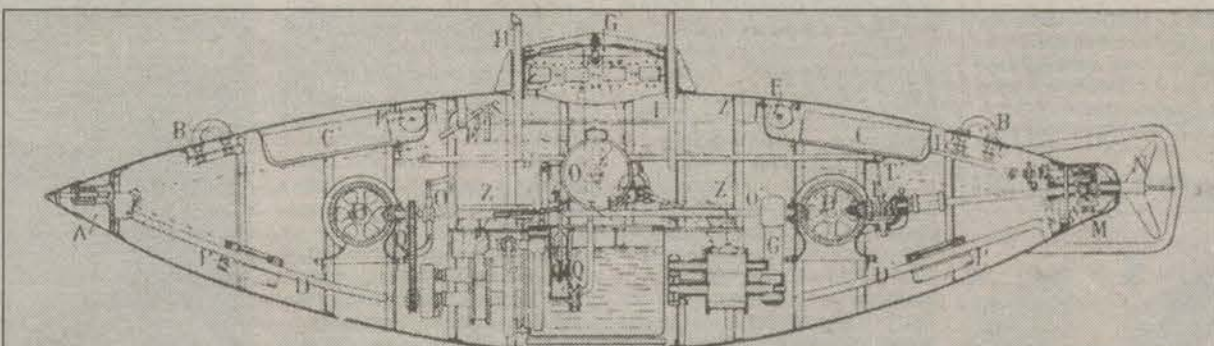
Чертеж подводной лодки Джевецкого (третий вариант), по которому была построена серия подводных лодок в количестве 50 единиц
